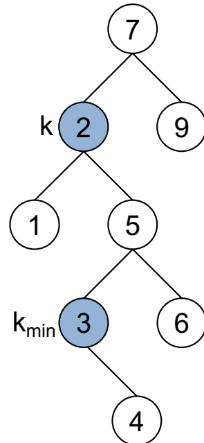
Suche kleinsten Knoten k_{\min} in rechten Teilbaum von k
